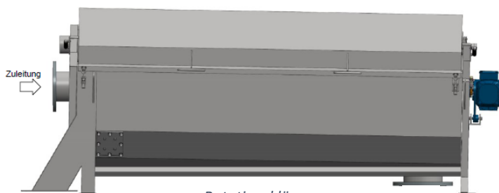
Rotationsklärer
