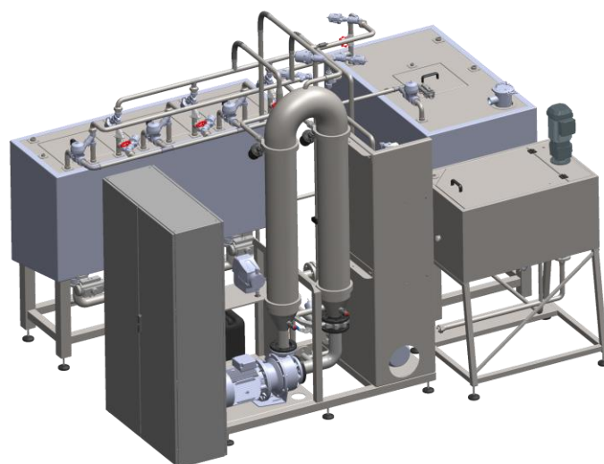
Schema Ultrafiltration mit Schwerkraftabscheider
